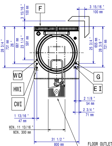
Boven aanzicht
